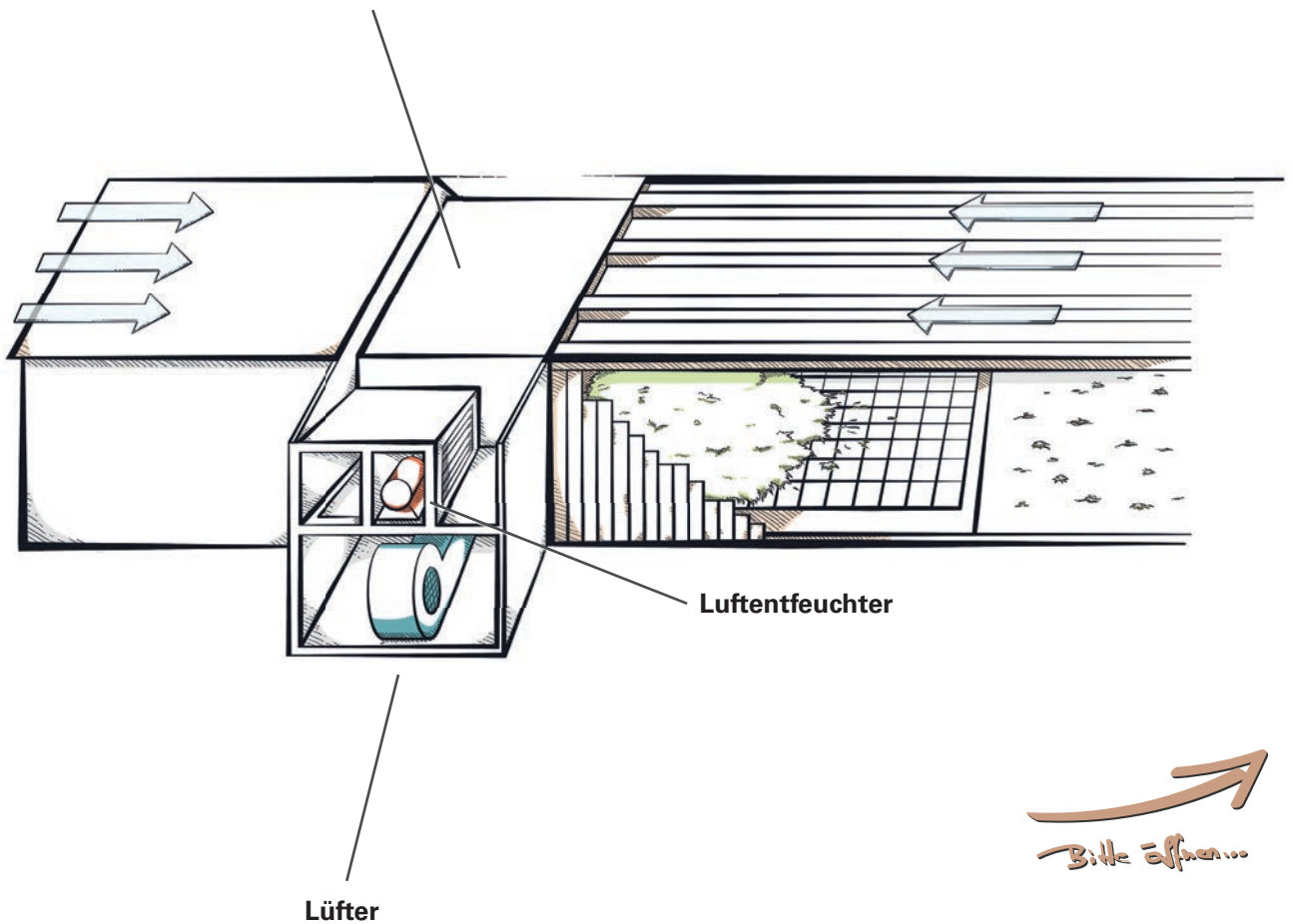
Dachabsaugung unter normalem Dach
